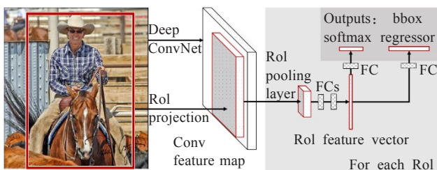
图9 Fast-R-CNN 网络结构
