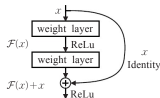
图7 残差单元
